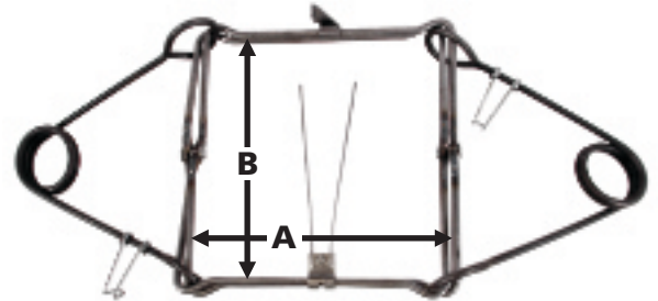
PIÈGE FERMÉ
