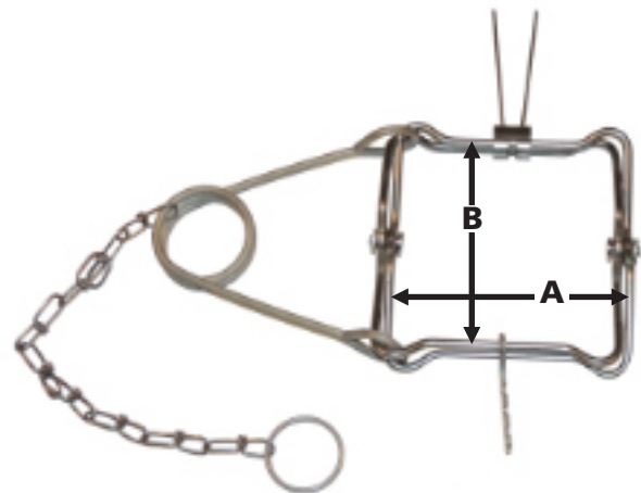
PIÈGE FERMÉ
